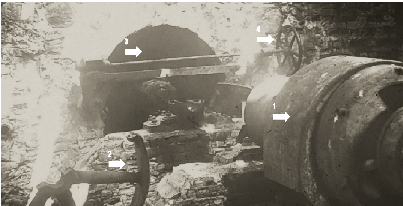
▲ Фота 256. Начынне электрастанцыі па спыненні яе працы: 1 – генератар; 2 – расшчэпленае кола раменнай перадачы для падвышэння хуткасці абаротаў; 3 – адтуліна выхаду вала турбіны; 4 – штурвал павароту лапатак турбіны для рэгулявання падачы вады. Каля 1973 г. Са збору І. Аўсюкевіча
